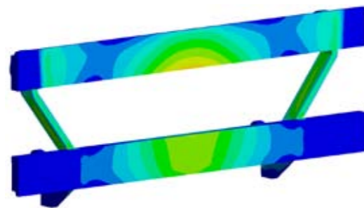
Spannungsoptimierte Konstruktion (Abbildung zeigt Finite Elemente Berechnung)
